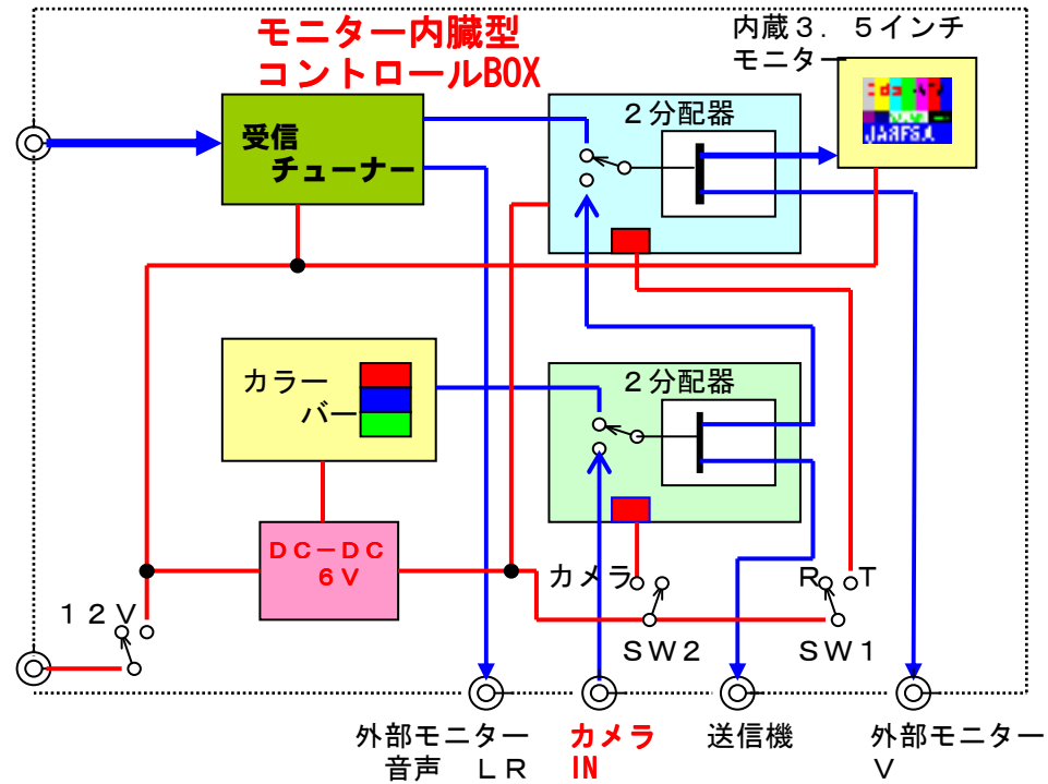
JA8FSA D-TV 構成図
